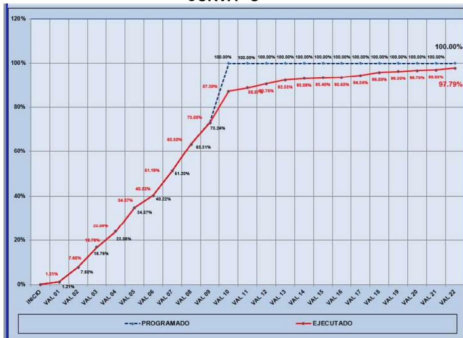
CURVA “S”
